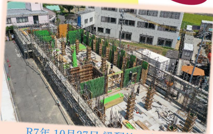
R7年10月27日 梁配筋工事中
